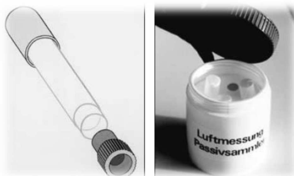
Figure 1 : tube passif et boîte de protection pour la mesure du \text{NO}_2
