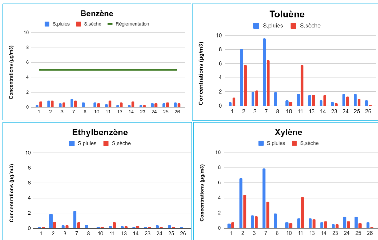
Figure 6 : Représentation des concentrations des BTEX
