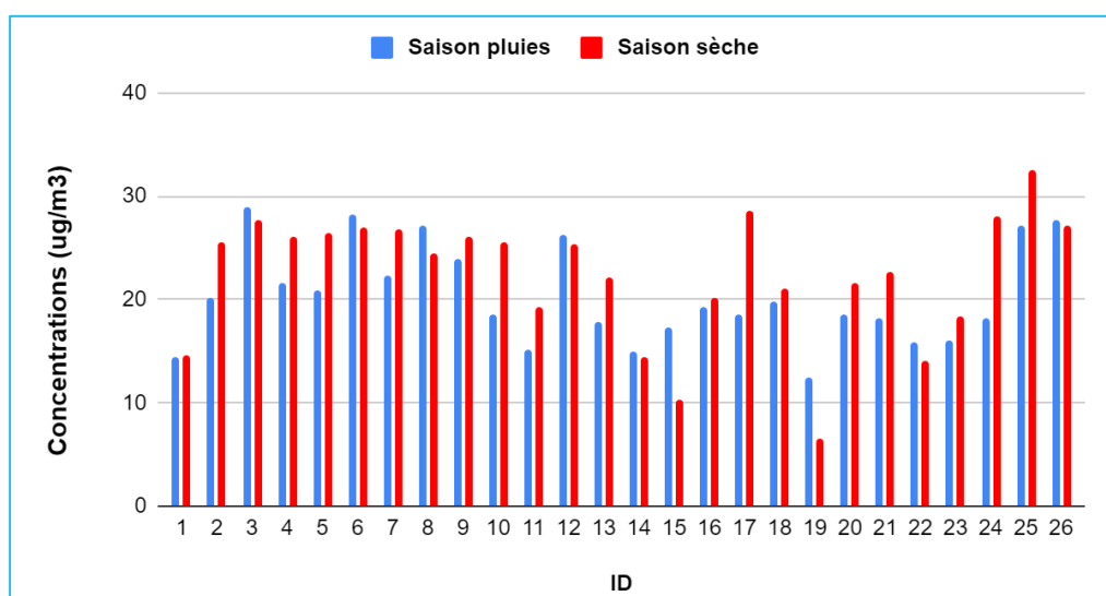
Figure 5 : Représentation des concentrations d'ozone
