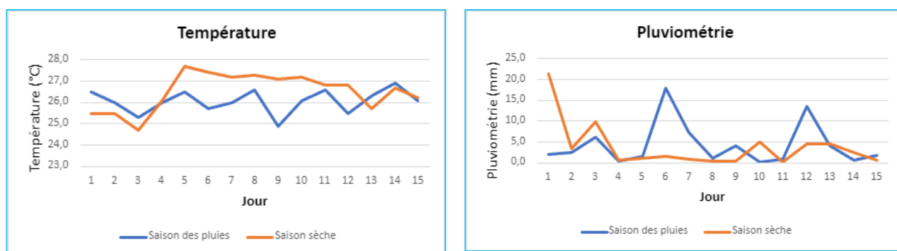
Figure 9 : Représentation de la pluviométrie et température durant les 2 campagnes
