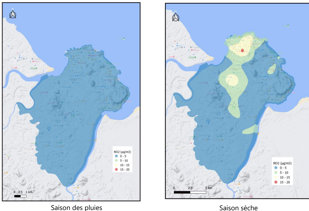
Figure 7 : Spatialisation du dioxyde d'azote sur l'île de Cayenne
