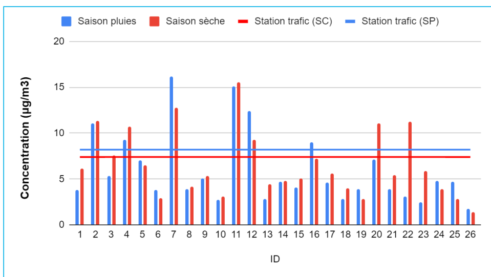
Figure 8 : Comparaison des concentrations du dioxyde d'azote avec les stations de mesure
